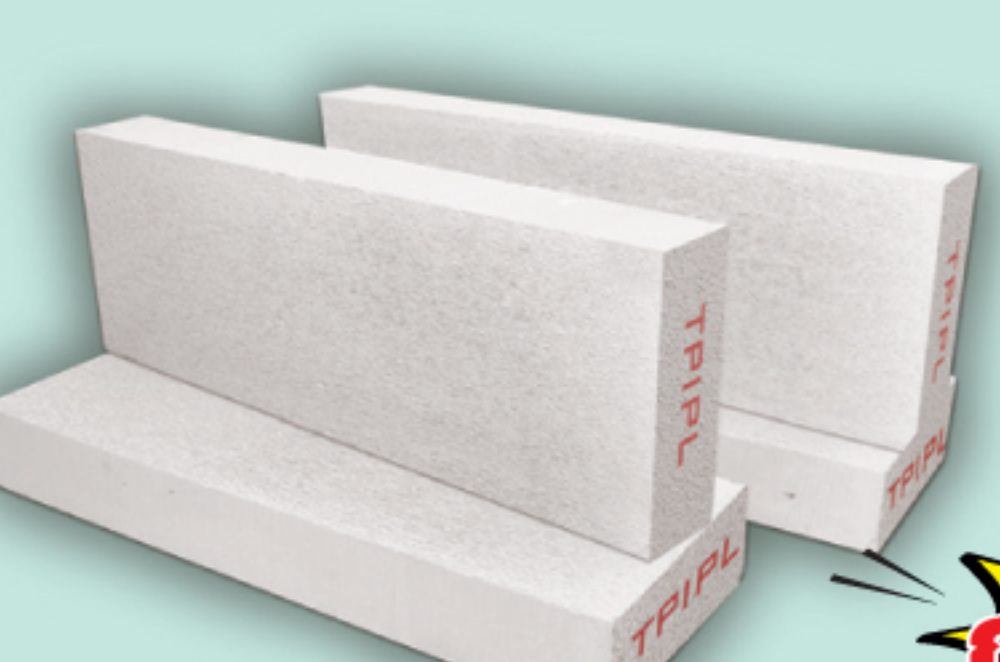
อิฐมวลเบา ขนาด 60x20x7.5 ซม.
